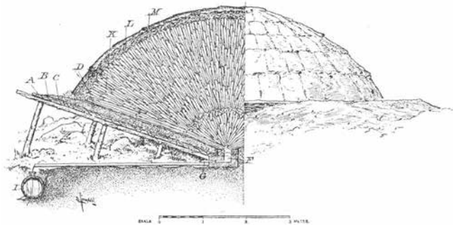
Pyöreä rännillinen tervahauta 1900-luvun alun ruotsalaisessa miilunpoltto-oppaassa.
